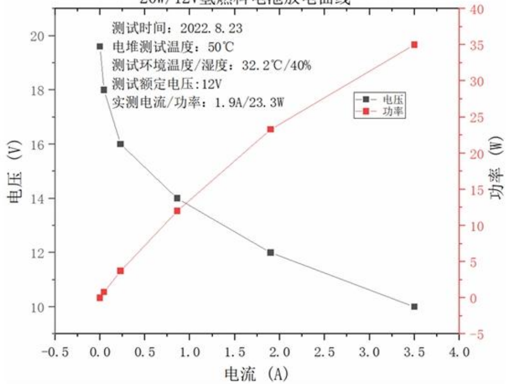
20W/12V氢燃料电池放电曲线
